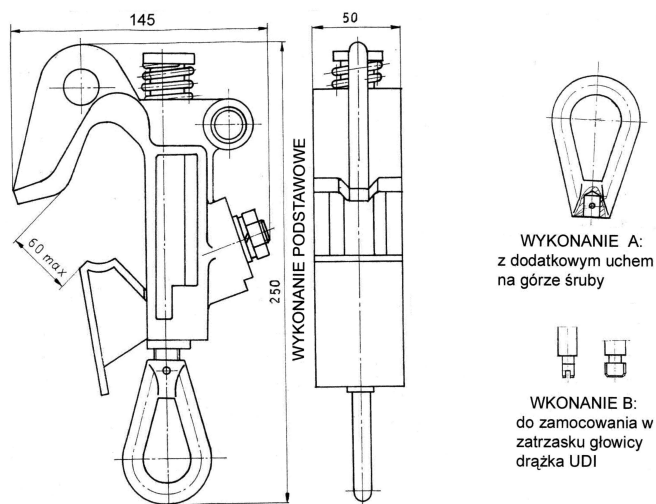
RYS.2 Zaciski ZF-3
