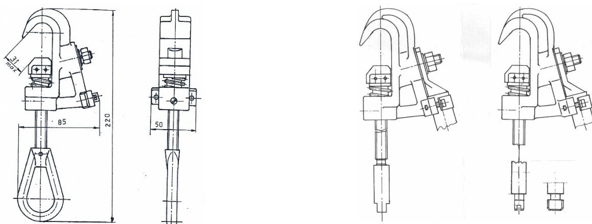
ZF-2 do przewodów okrągłych wykonanie podstawowe
